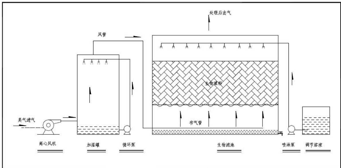
图 6.2-2 生物滤池工艺流程图
